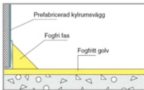
Bild 3.4: Anslutning mot prefabricerad kylrumsvägg. Fas: bredd 20-30 mm, höjd 20-30 mm.
